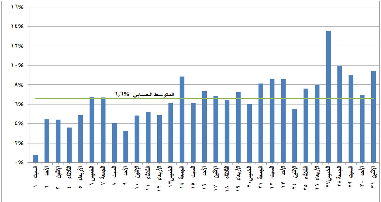
شكل (٩) النسب المئوية للتغير في الحمل الاقصى خلال شهر يناير ٢٠٢٢ مقارنة باليوم المماثل من العام الماضي
