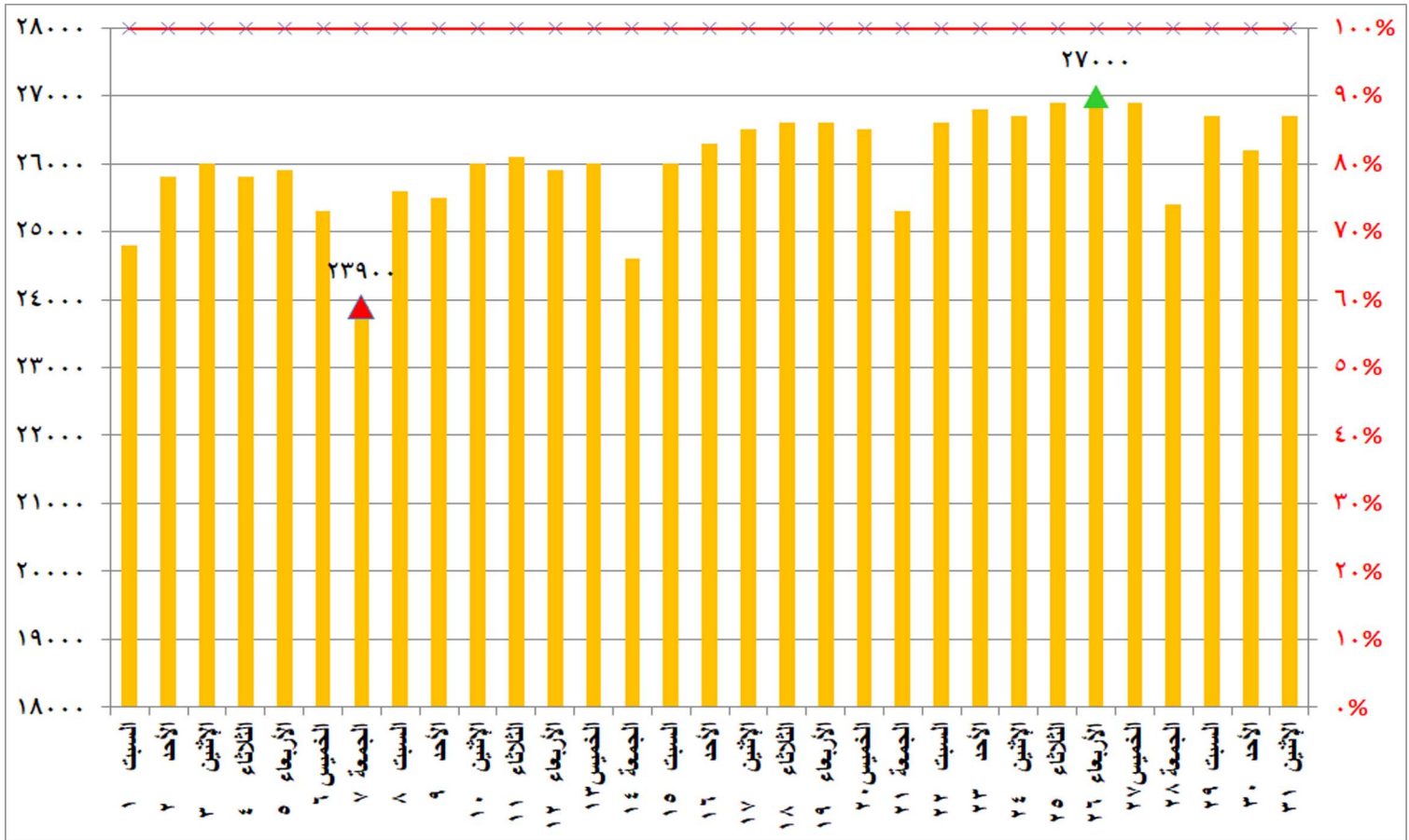
شكل (٥) قدرات الانتاج المتاحة ونسبتها للحمل الاقصى خلال شهر يناير ٢٠٢٢
