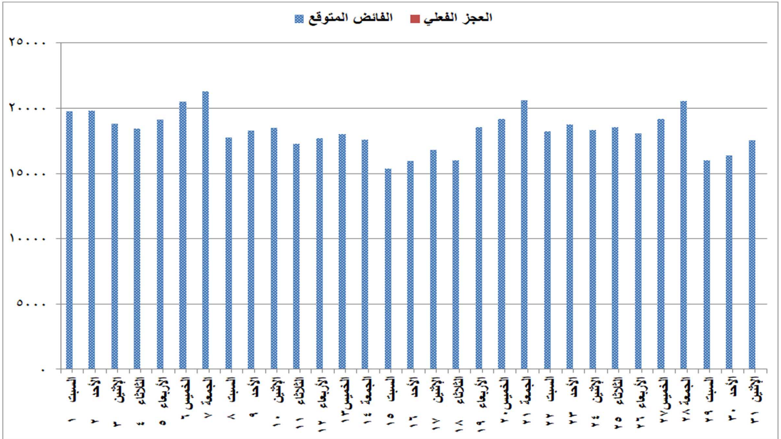
شكل (٧) الفااض والعجز المتوقع للقدرات خلال شهر يناير ٢٠٢٢
