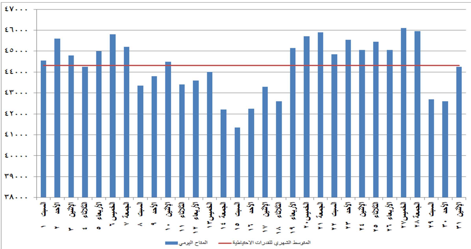
شكل (٢٧) القدرات المتاحة يوميا والمتوسط الشهري للقدرات الاحتياطية خلال شهر يناير ٢٠٢٢
