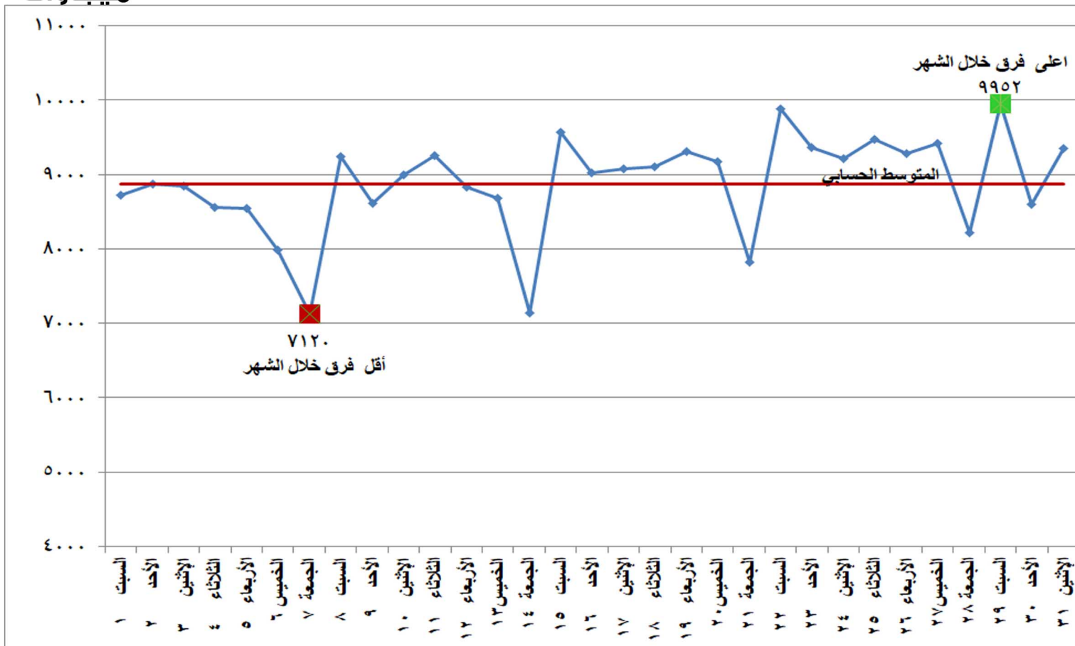
شكل (٣) الفرق بين أقصى وأدنى حمل خلال شهر يناير ٢٠٢٢
