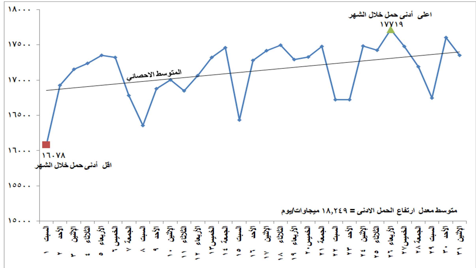
شكل (٢) تطور الحمل الأدنى اليومي خلال شهر يناير ٢٠٢٢
