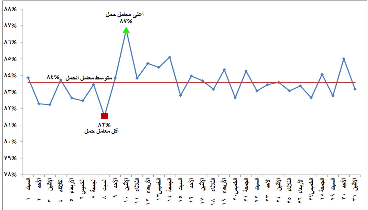
شكل (١٢) إجمالي معامل الحمل لوحدات الانتاج خلال شهر يناير ٢٠٢٢
