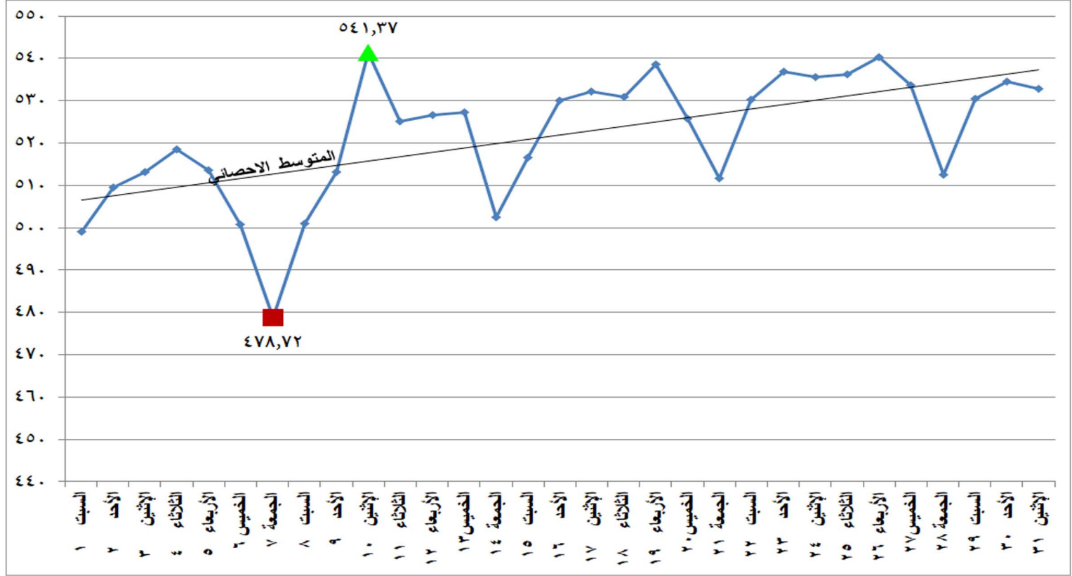
شكل (١٥) إجمالي الطاقة الكهربائية المنتجة من كل المصادر الأولية خلال شهر يناير ٢٠٢٢
