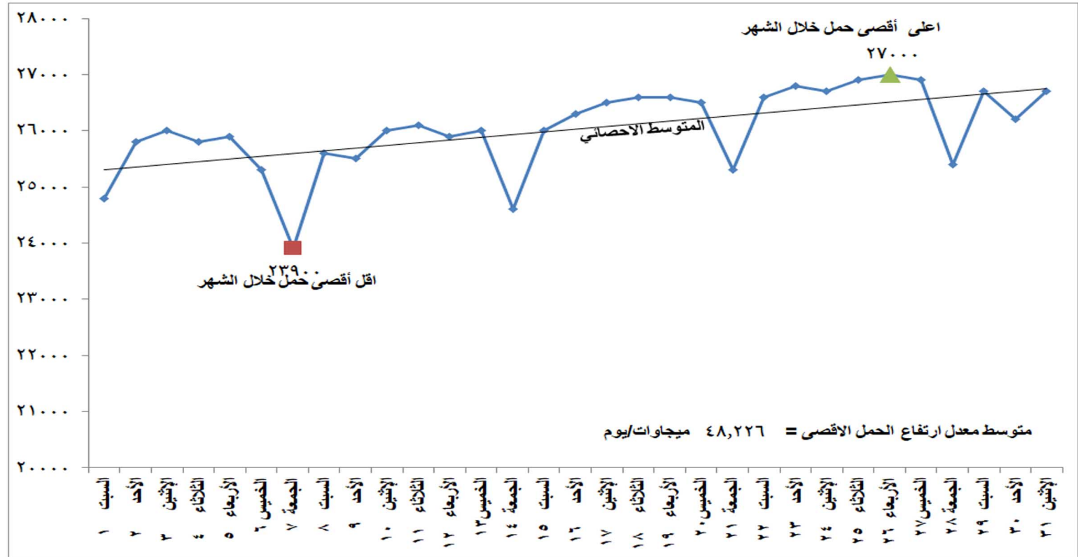
شكل (١) تطور الحمل الاقصى اليومي خلال شهر يناير ٢٠٢٢
