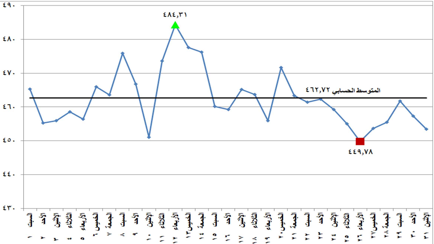
شكل (١٤) معامل انبعاثات غاز ثاني اكسيد الكربون المكافئ على مدى شهر يناير ٢٠٢٢
