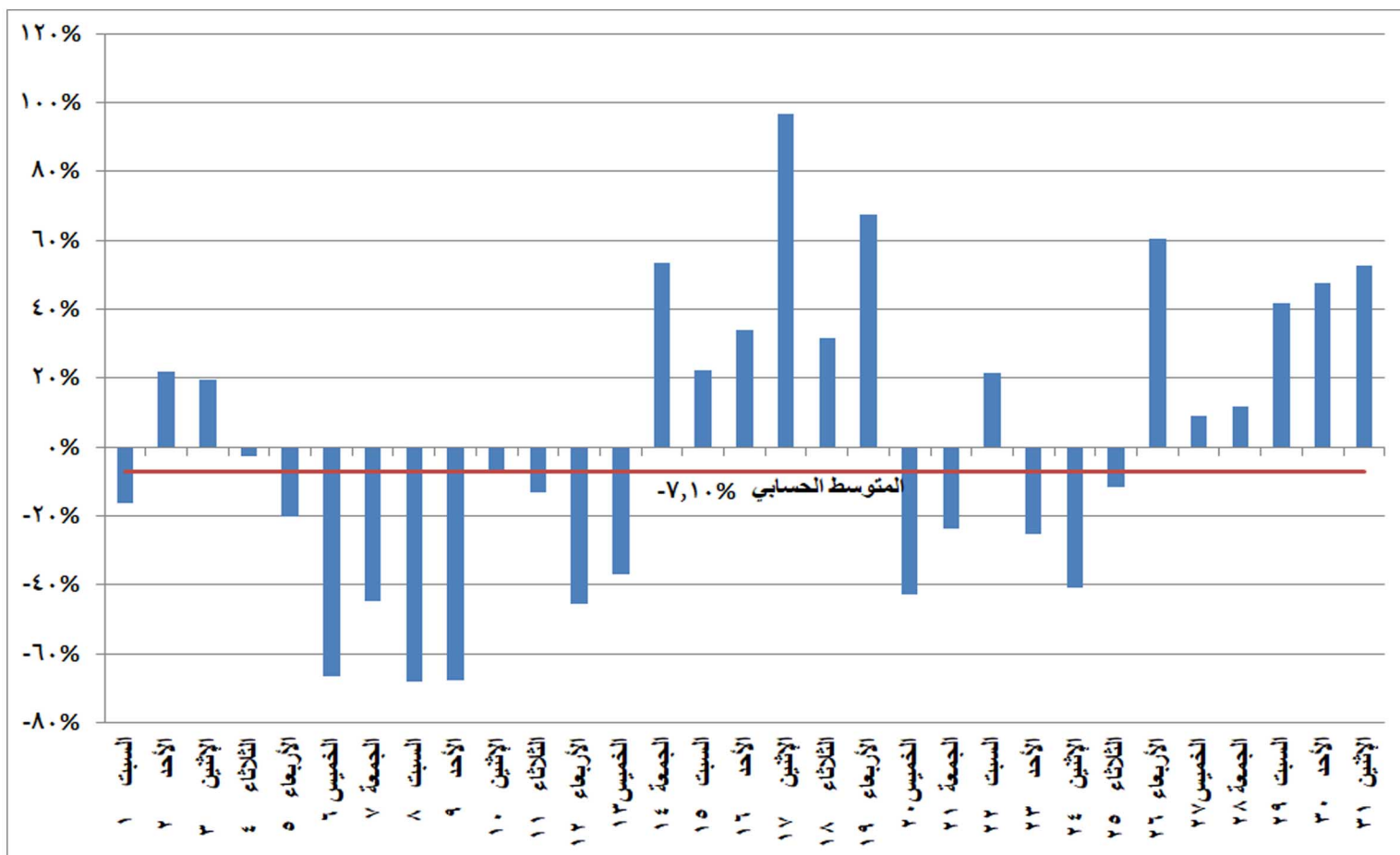
شكل (٢٦) نسب التغير في استخدام الرياح والشمس في إنتاج الطاقة الكهربائية خلال شهر يناير ٢٠٢٢ مقارنة بالشهر المماثل من العام السابق
