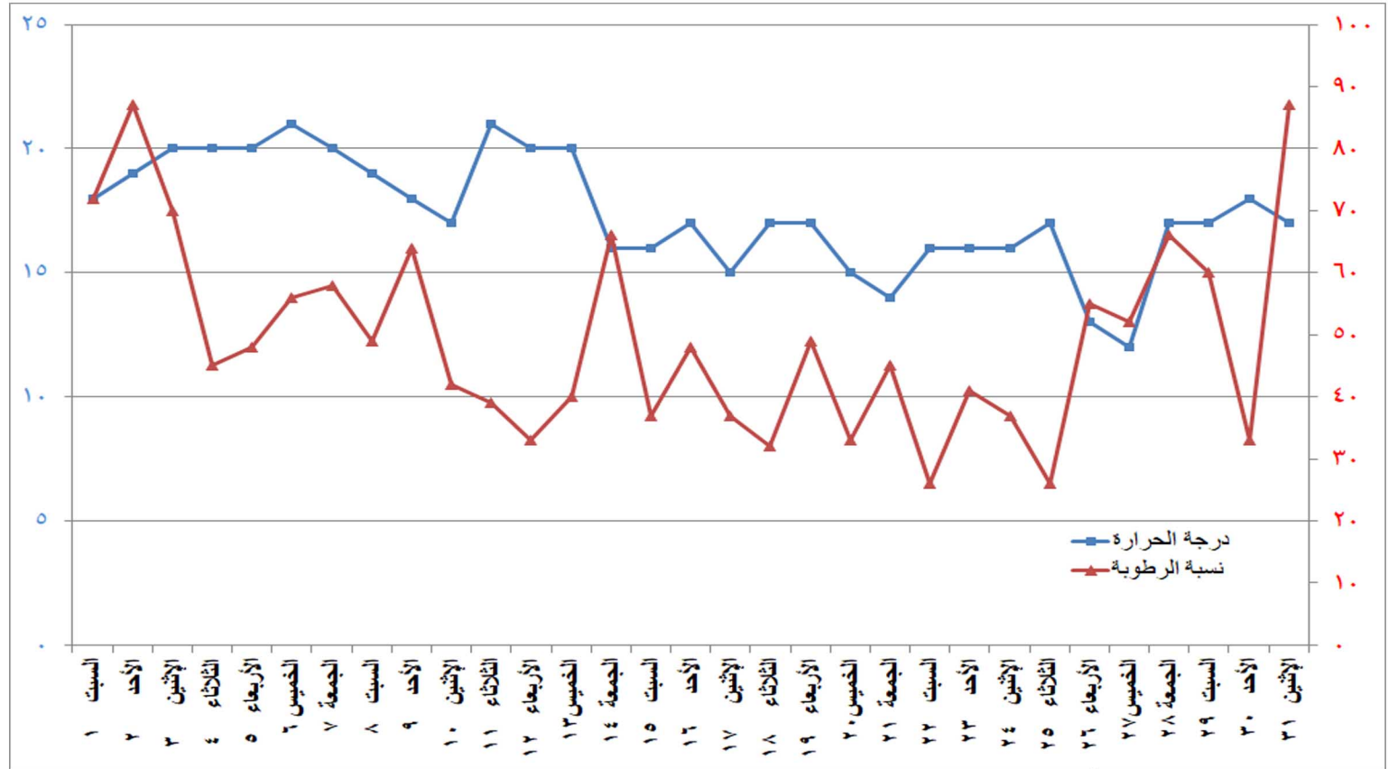
شكل (١١) التغيير في درجة الحرارة والرطوبة النسبية خلال شهر يناير ٢٠٢٢
