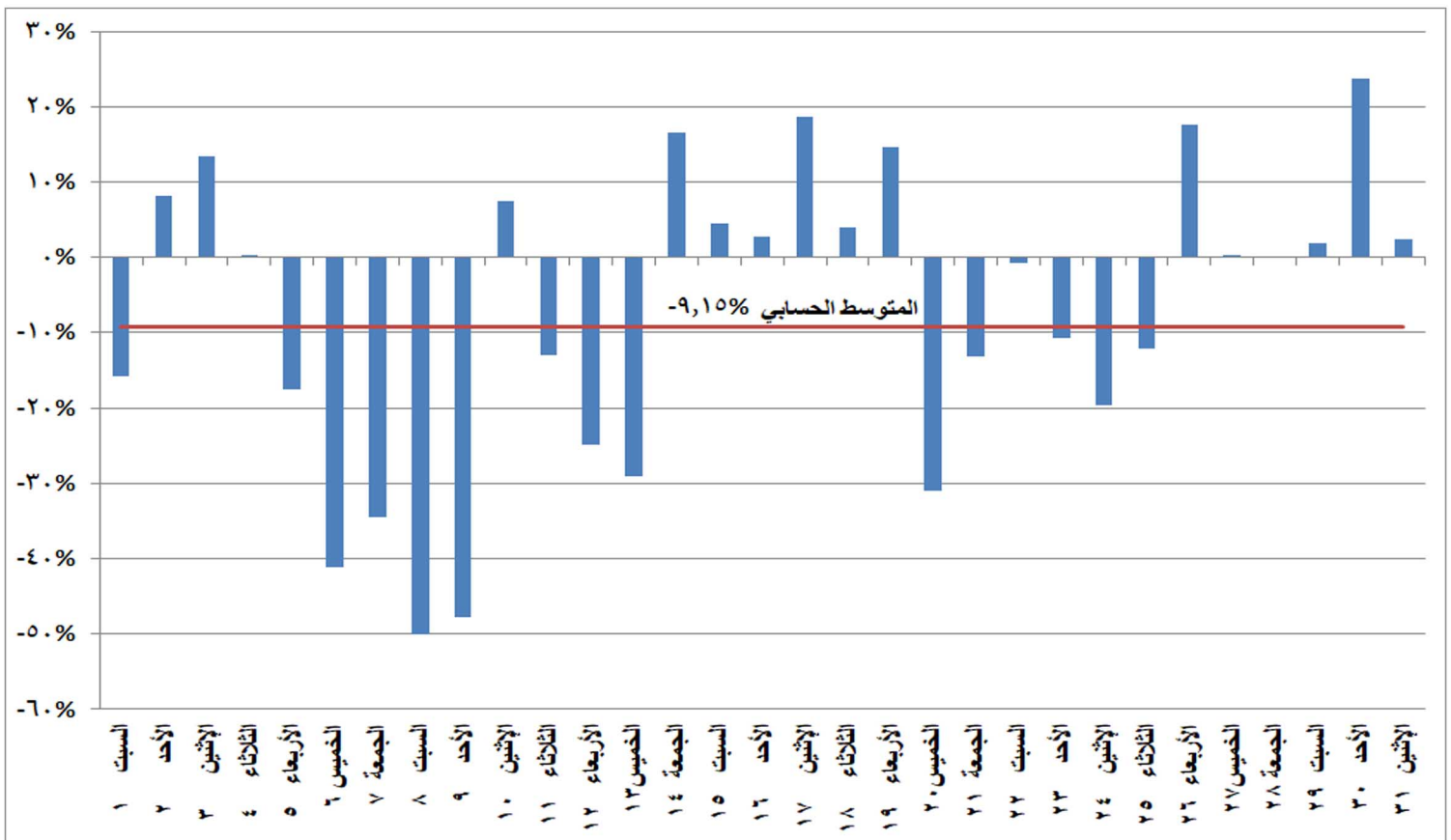
شكل (٢٢) نسب التغير في استخدام المصادر غير الحرارية في إنتاج الطاقة الكهربائية خلال شهر يناير ٢٠٢٢ مقارنة بالشهر المماثل من العام السابق
