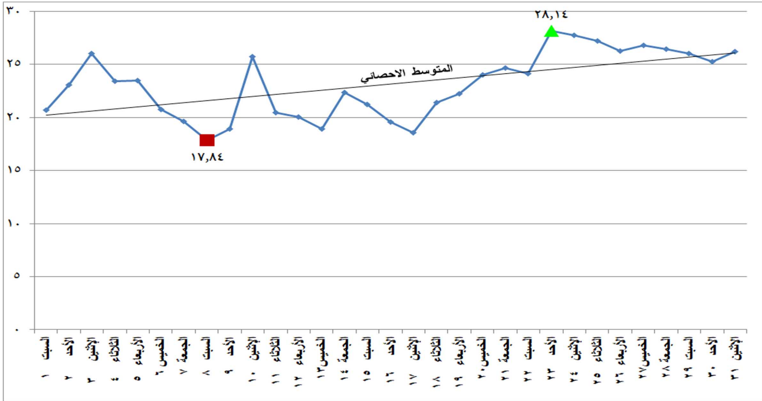
شكل (٢٣) الطاقة الكهربائية المنتجة من المصادر المائية خلال شهر يناير ٢٠٢٢
