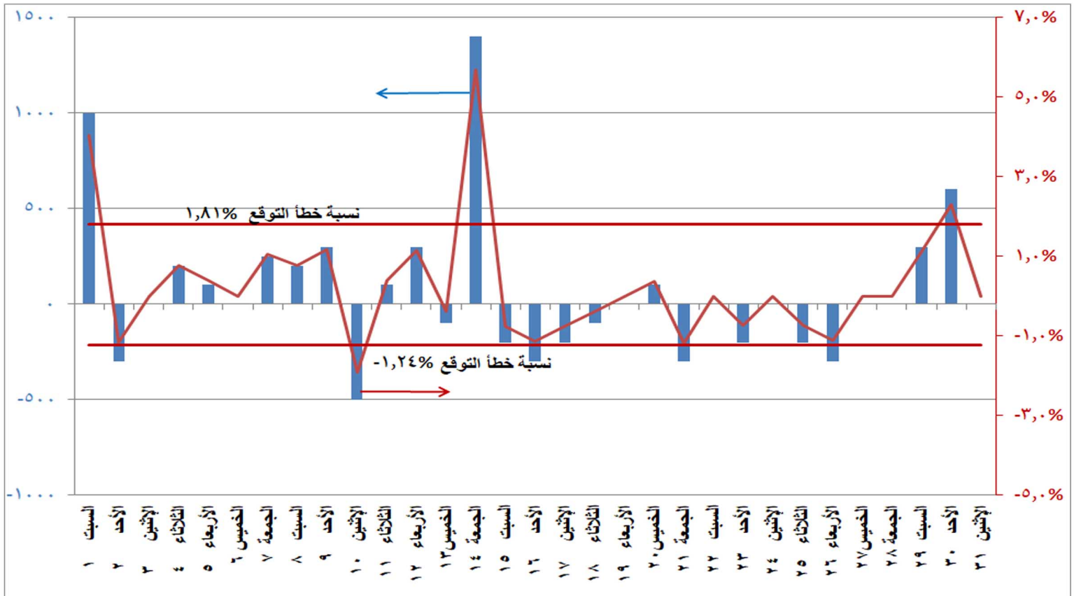
شكل (١٠) الفرق بين الحمل الأقصى المتوقع والمسجل فعليا ونسبة الفرق إلى الحمل المسجل فعليا خلال شهر يناير ٢٠٢٢
