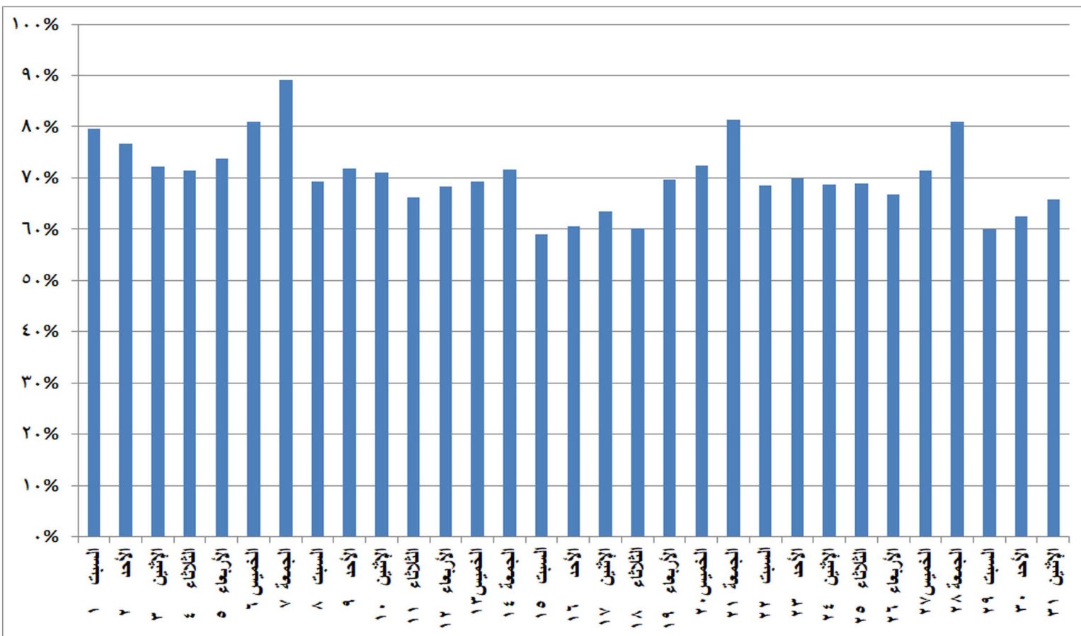
شكل (٢٨) نسب الفائض للحمل الاقصى المسجل يوميا خلال شهر يناير ٢٠٢٢
