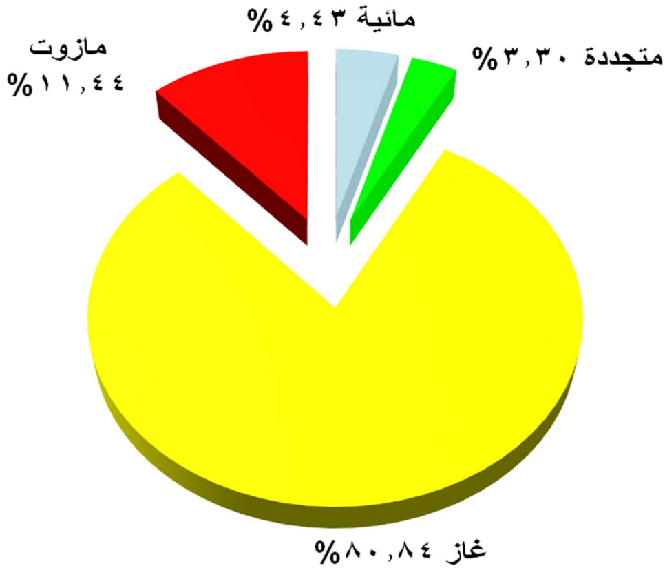
شكل (١٣) متوسط نسب مشاركة مصادر الطاقة الاولية في انتاج الكهرباء خلال شهر يناير ٢٠٢٢
